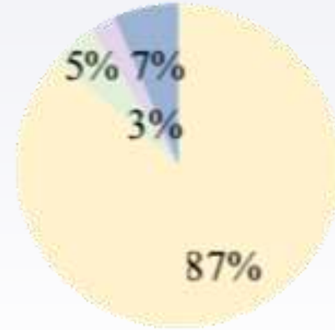
LLaMA (65B)
