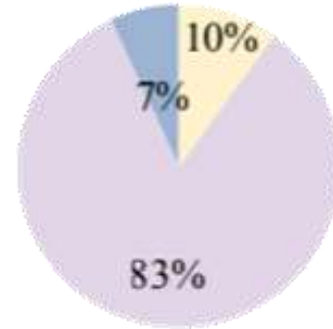
Galactica (120B)
