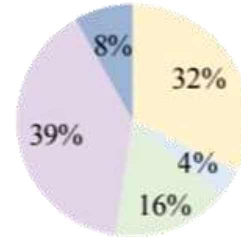
GPT-NeoX (20B)
