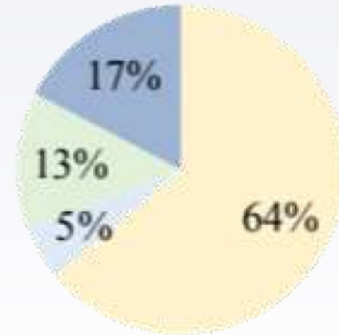
GPT-3 (175B)
